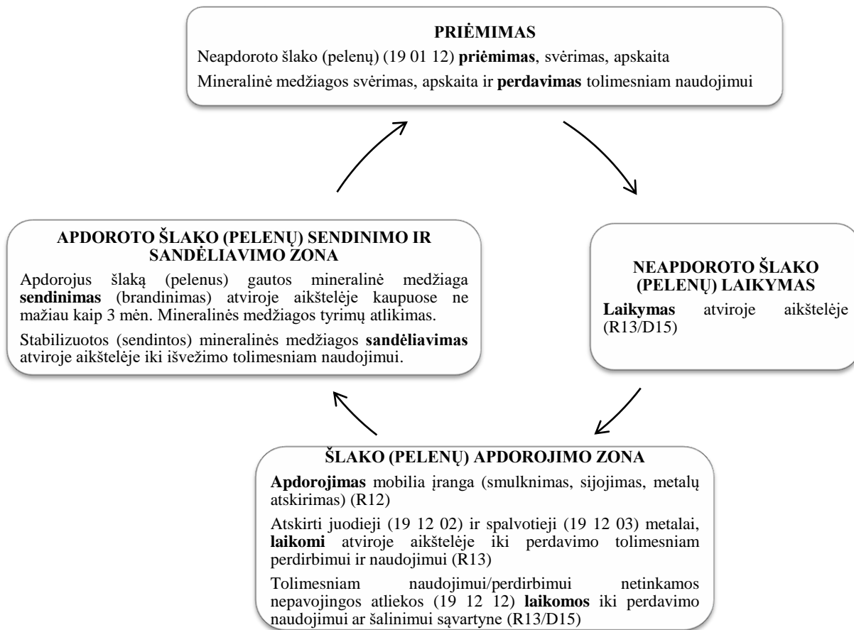
2 pav. PUV nepavojingų pelenų (šlako) laikymo ir apdorojimo aikštelėje principinė technologinė schema
